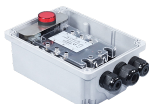
Aluminiumgehäuse mit 3-poligen Halbleiterrelais, Temperaturalarm und Alarm-Blinkleuchte.
